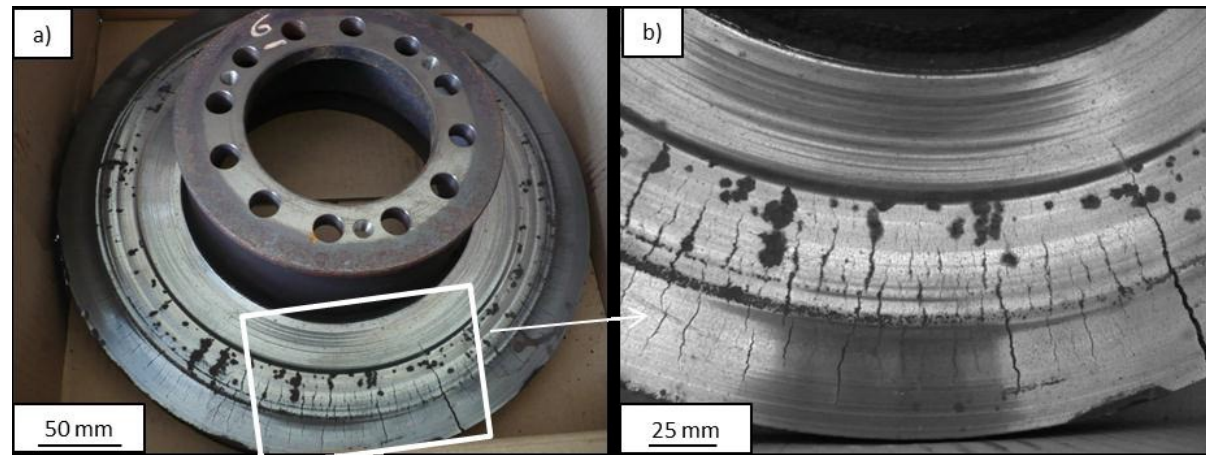
Ex: disque de frein de poids lourds (source: CTIF)
